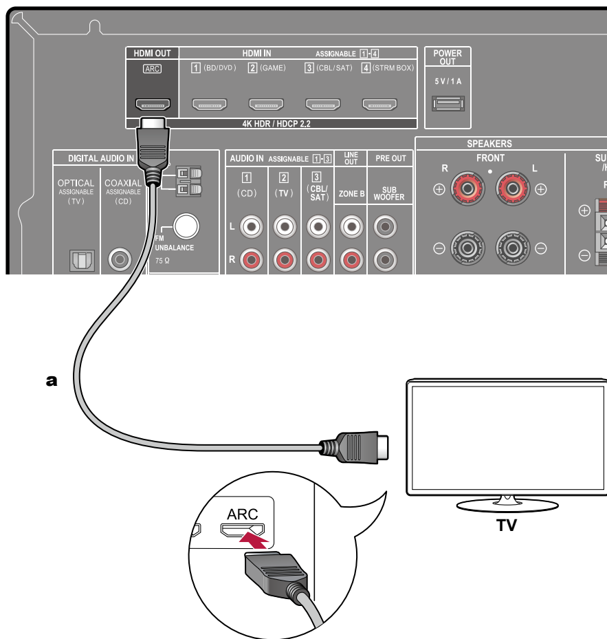
a HDMI-kabel
